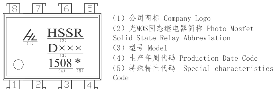
图 5 产品印章 Figure 5- Marking
