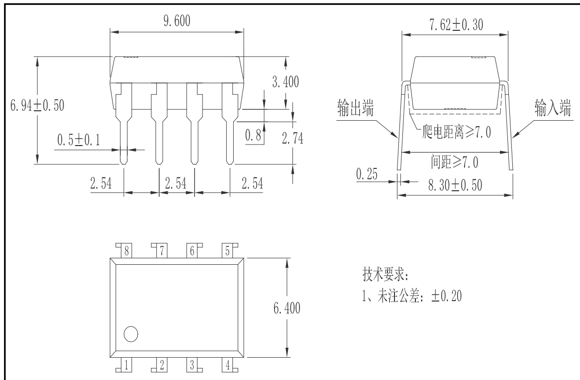
图 3 HSSR-DA08 外形尺寸
