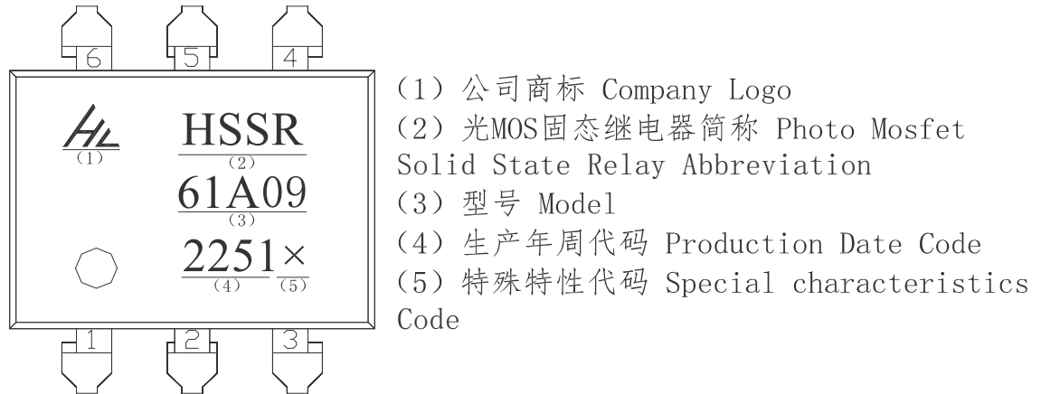
图 10 产品印章 Figure 10- Marking
