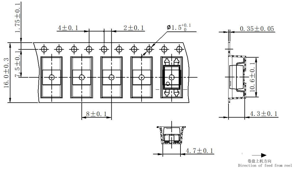
卷盘外形图 Reel's Dimensions
