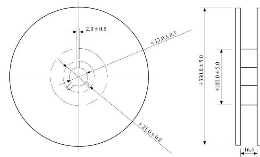
卷盘外形图 Reel's Dimensions
