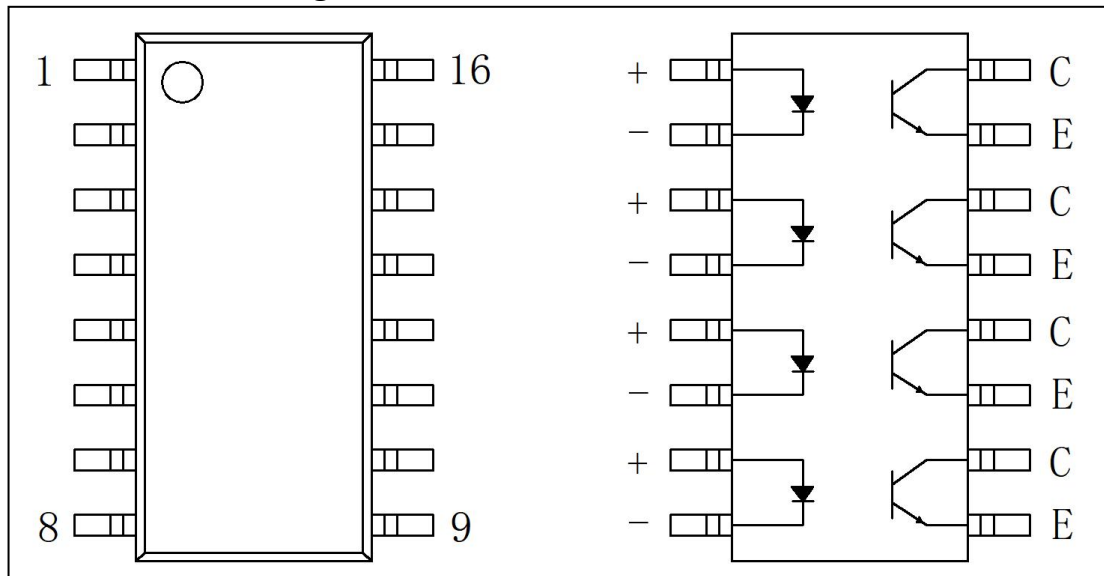
图 3 电原理图 Figure 3-Schematic
