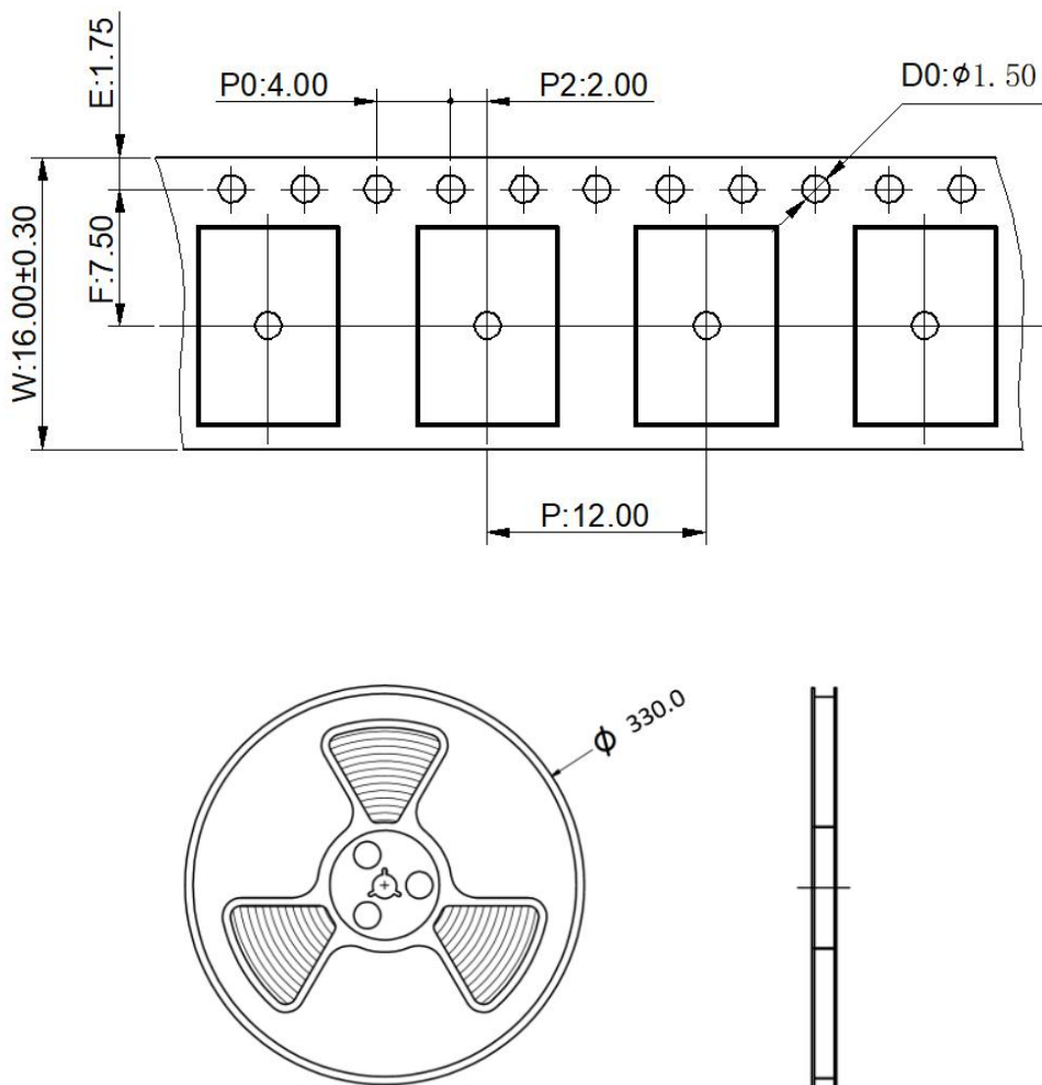
图 6 编带包装示意图
