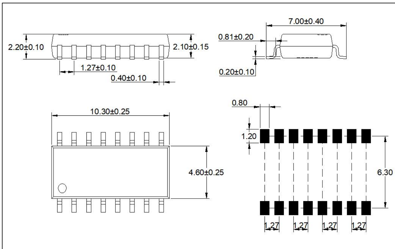
图 4 HPC247× 外形尺寸
