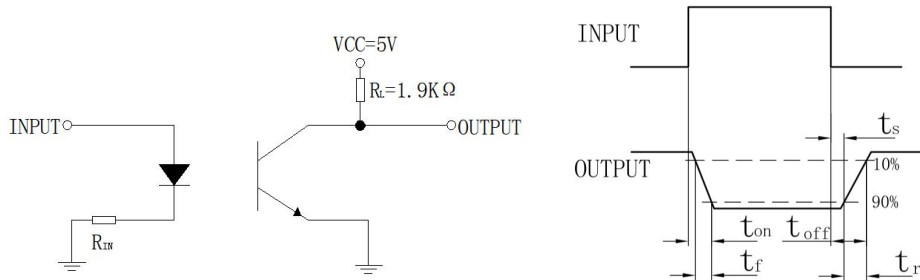
图 2 t_{on} , t_s , t_{off} 测试方法 Figure 2- The test method of t_{on} , t_s , t_{off}
